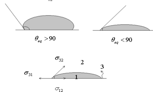
Fig. 2. Contact angle.
