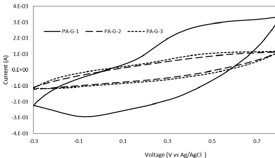
Fig. 1. Cyclic voltammograms
